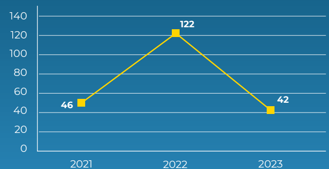
PSV (€/MWh)
